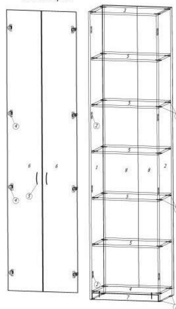
Схема сборки
