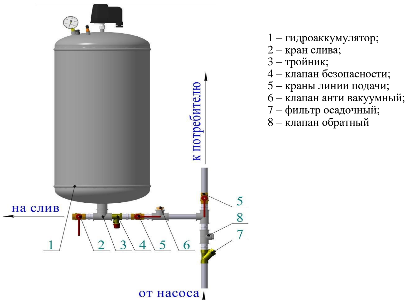
Рисунок 3 – Условная схема подключения гидроаккумулятора к водопроводным сетям жилого дома
