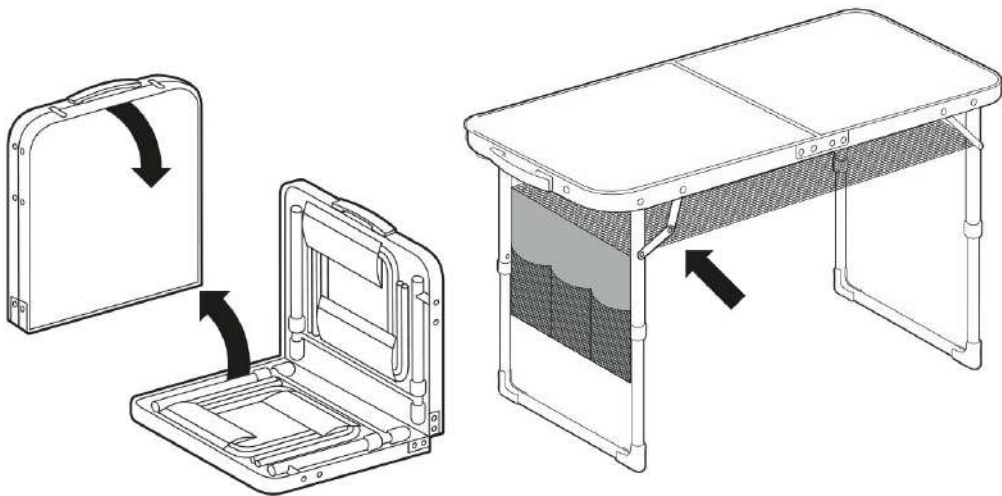
(рис. 3) Схема установки стола
