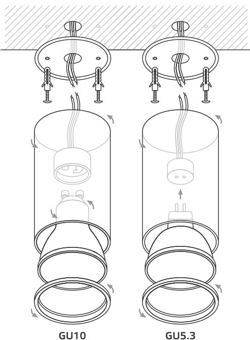
Рис. 2. Порядок монтажа.
