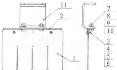
Рисунок 6 – Установка шторы на моторблоки: «Салют», «Авангард».
