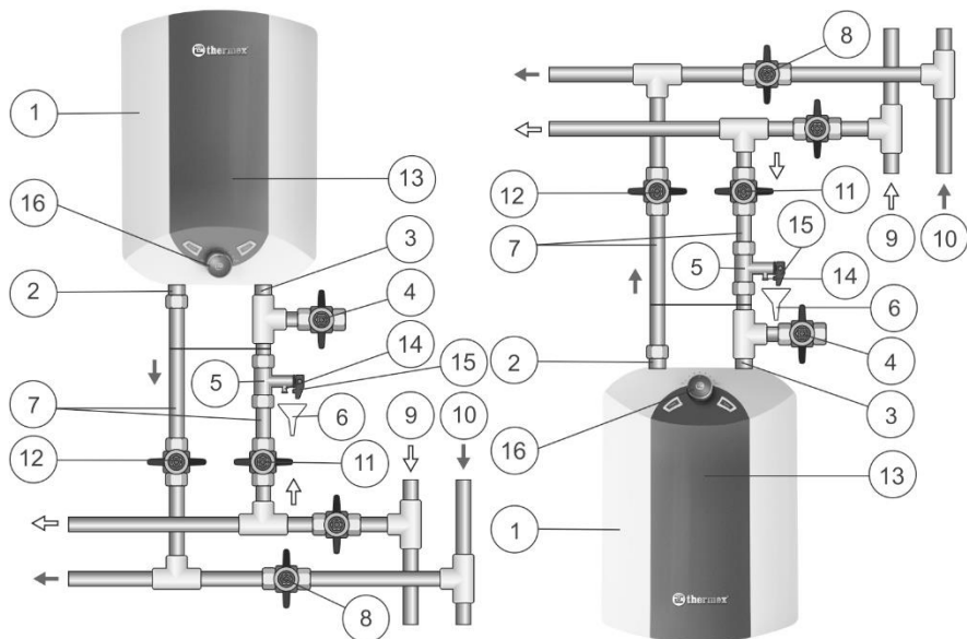
Рисунок 2. Схема подключения ЭВН к водопроводу моделей Galaxy 15 О (слева) и Galaxy 15 U (справа):
