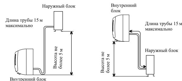
Схема установки
